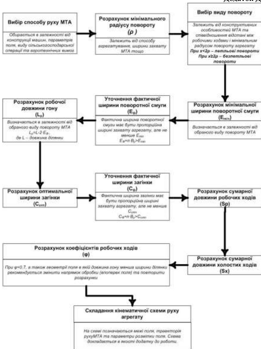
Рис. Д.1. Схема кінематичного розрахунку МТА
