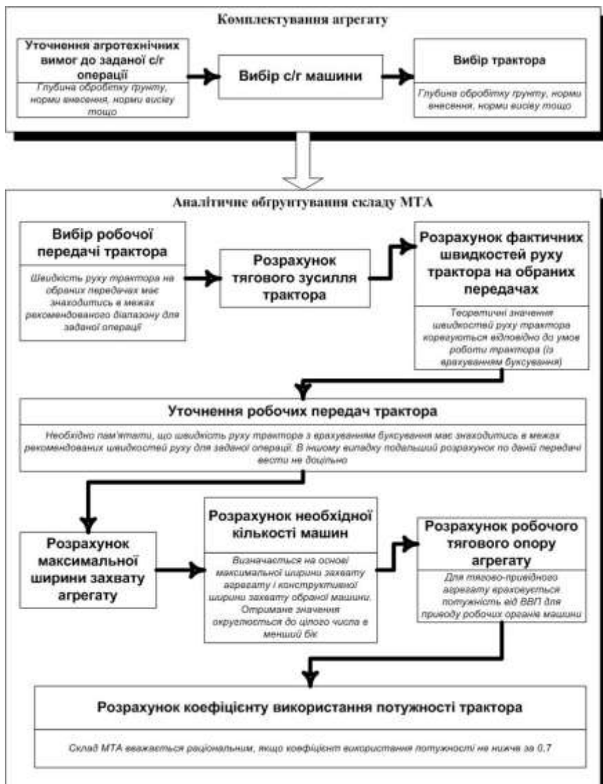
Рис. Г.1. Схема тягового розрахунку МТА
