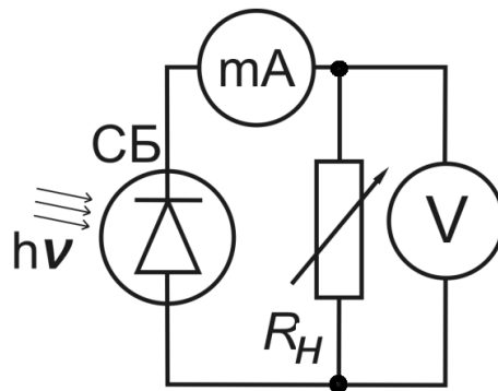
Рис. 6. Схема експериментальної установки
