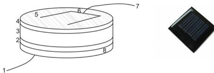
Рис. 1. Типова структура сонячного елемента з p-n -переходом (скляна і пластикова кришка елемента і фільтр між елементом і кришкою не зображені) та сонячний модуль УН 40×40-4А/В40-Р
