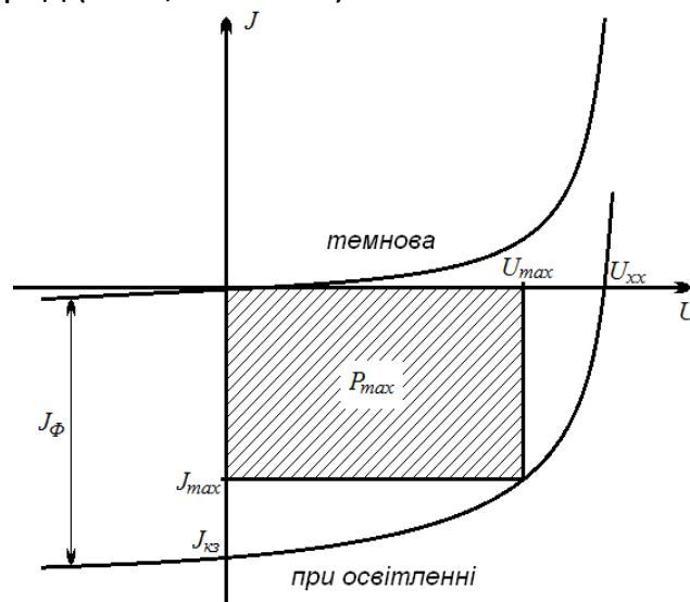
Рис. 5. ВАХ сонячного елемента в темряві і при освітленні. U_{xx} – напруга холостого ходу (розмикання), J_{кз} – струм короткого замикання контактів у колі без участі опору навантаження; J_\phi – зворотний фотострум
